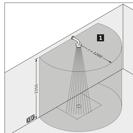
Situación en espacio de ducha sin plato (obra) o con plato de ducha enrasado
