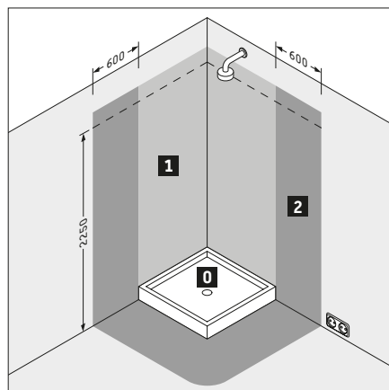
Situación en espacio con plato de ducha
